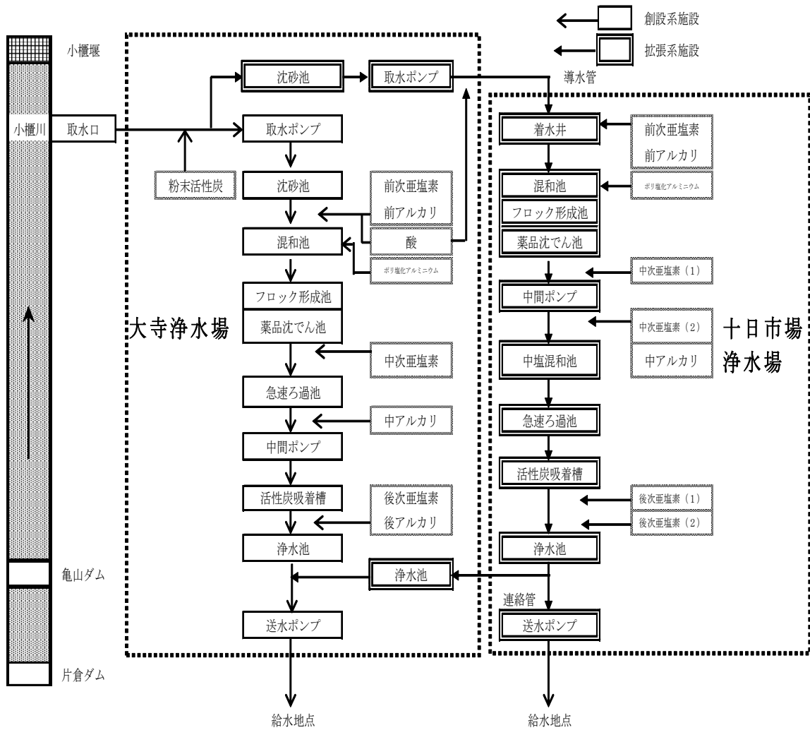
図-1 各浄水場フロー図
